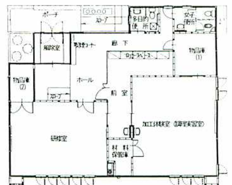
施設平面図
