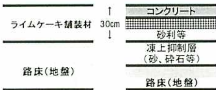
図1 舗装の構造
